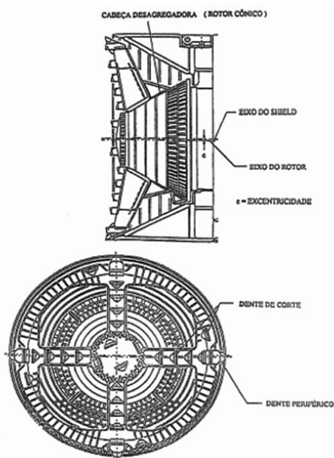
Figura 89 – Cabeça cortante desagregadora
