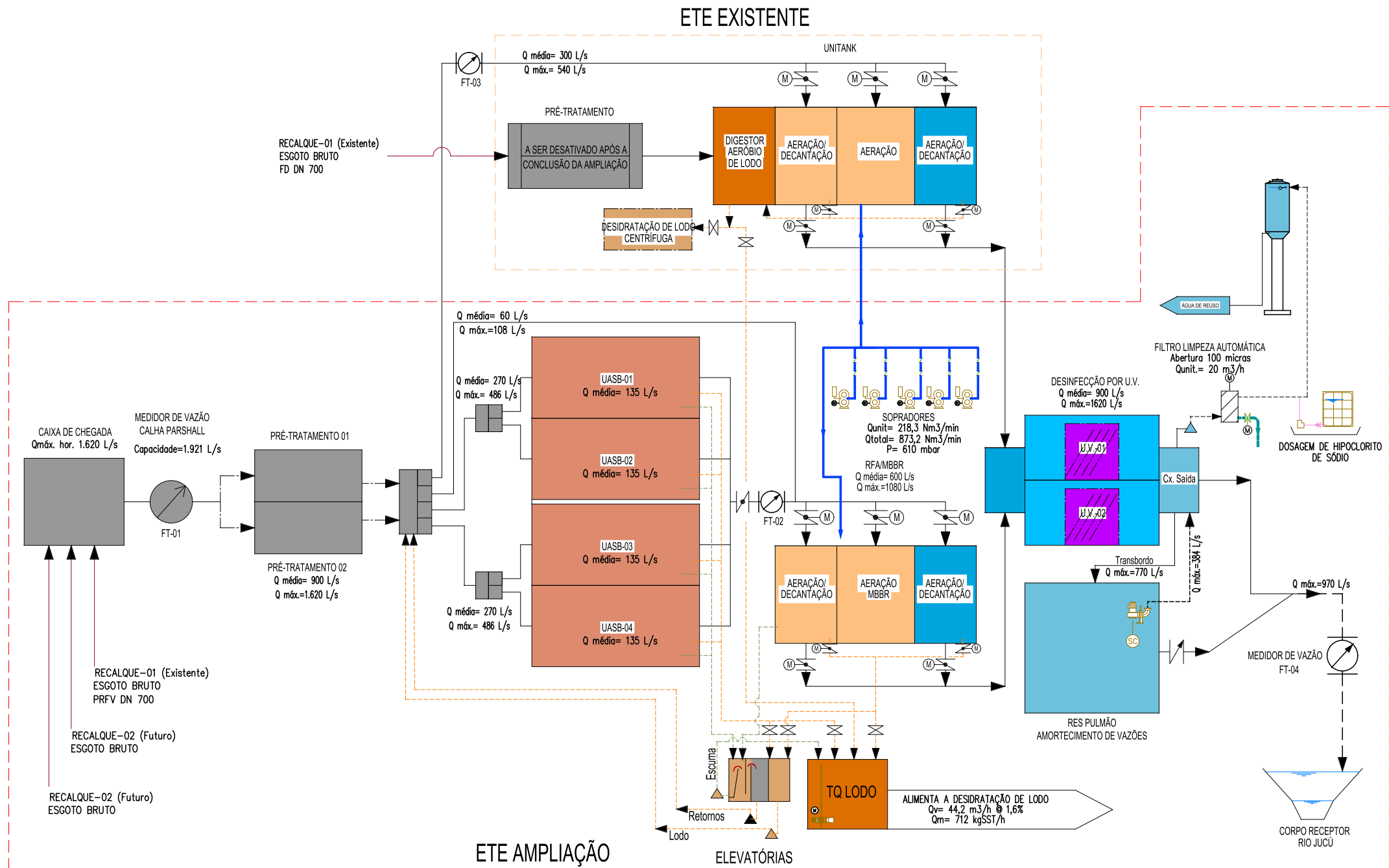
Figura xxx: Fluxograma ETE ARAÇAS - Fase Líquida
