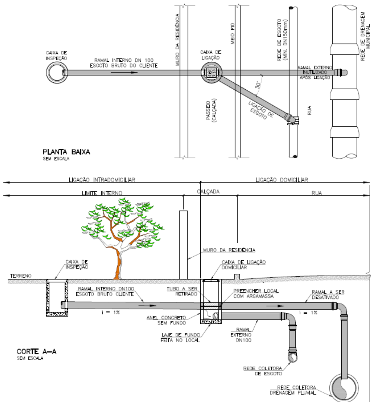
Figura 21 - Planta e corte da ligação domiciliar.
