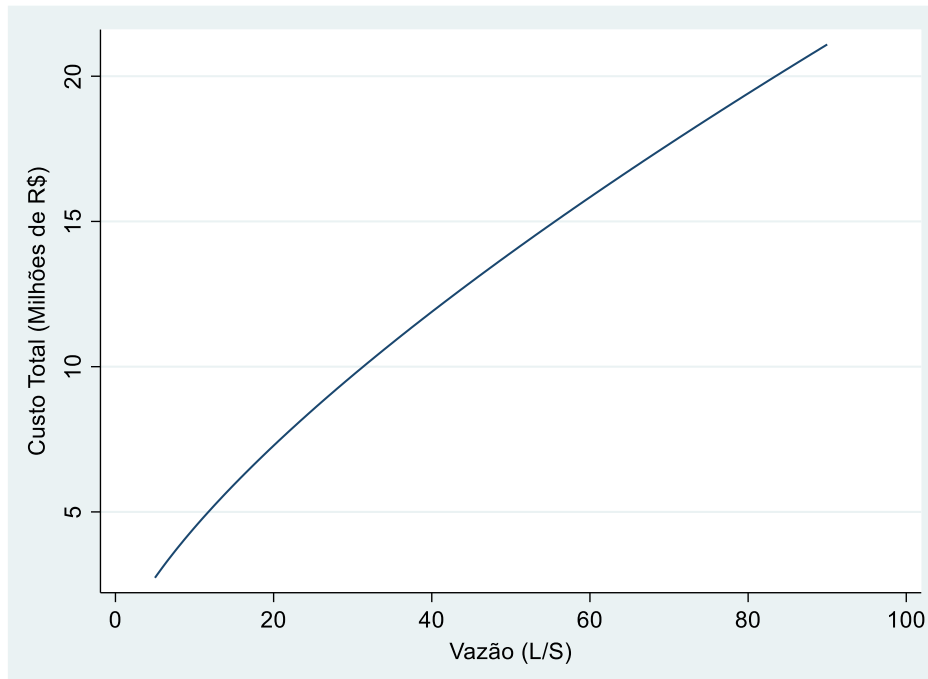
Figura 10 Curva de Custo x Vazão
