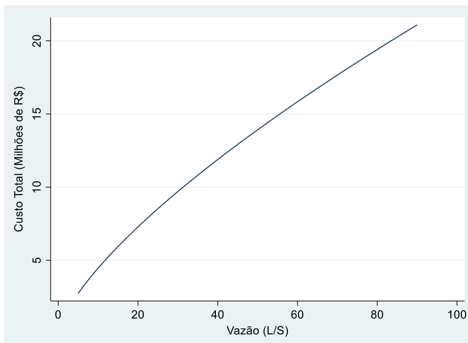
Figura 7 Curva de Custo x Vazão
