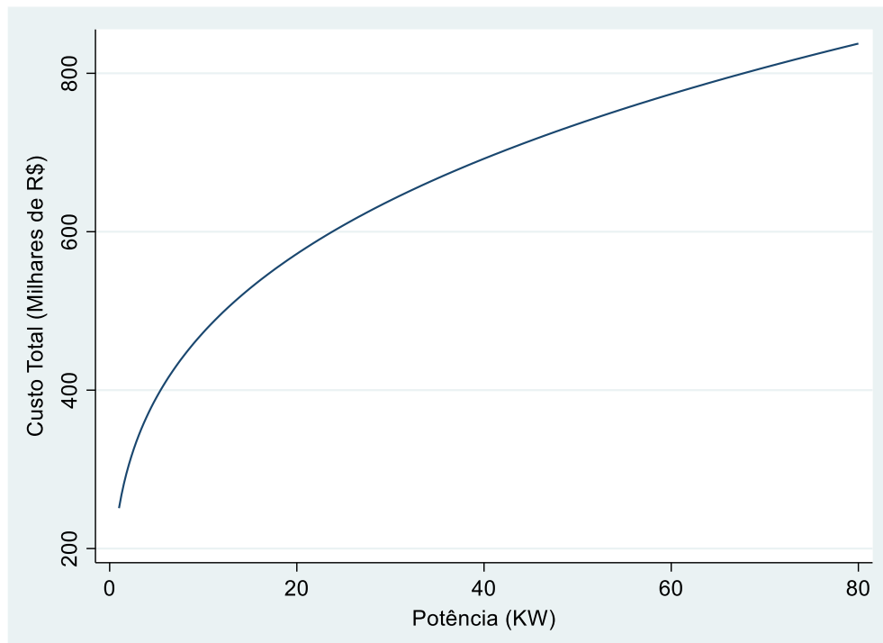
Figura 6 Curva de Custo x Potência
