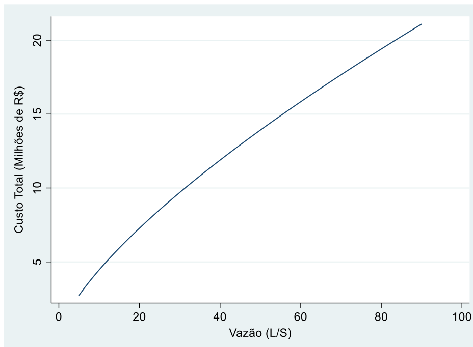
Figura 6 Curva de Custo x Vazão
